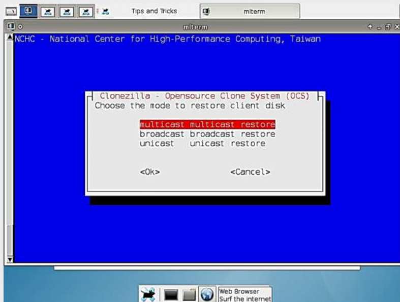
Fig. 3.80. Seleccionamos el modo a clonar nuestro disco
