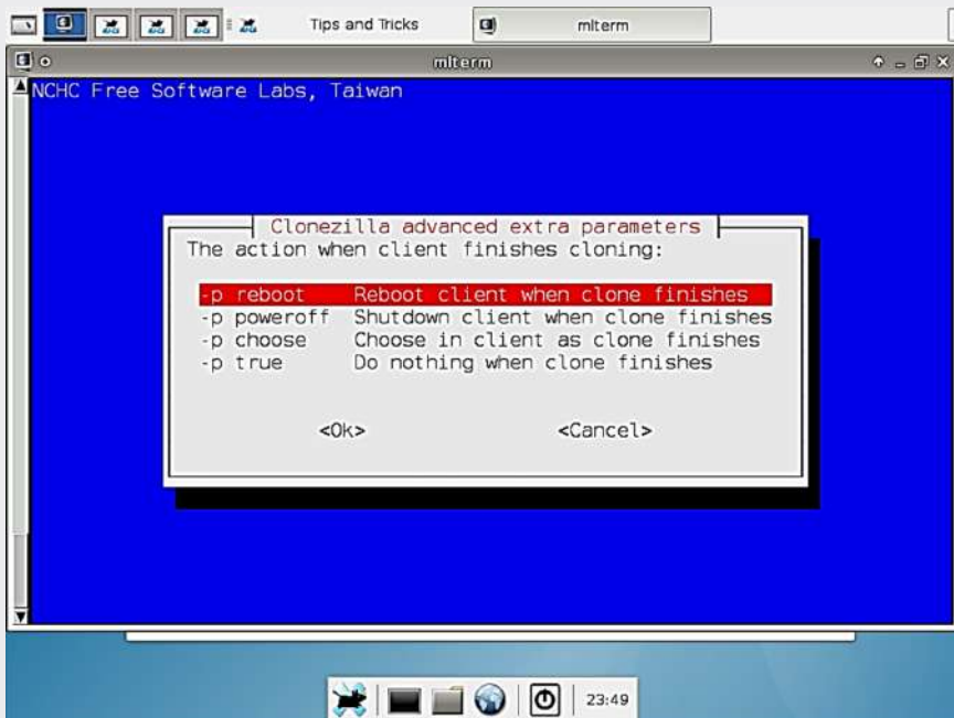
Fig. 3.77. Reinicio cuando termine la clonación
