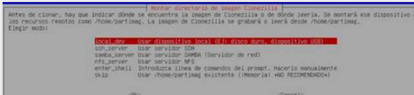
Fig. 3.34. Opciones de clonezilla para clonar el disco
