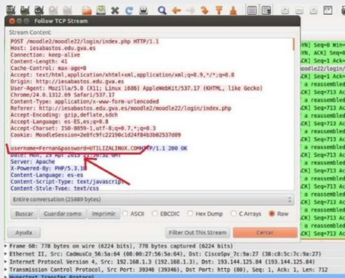
Fig. 3.13. Podemos observar el login y contraseña
