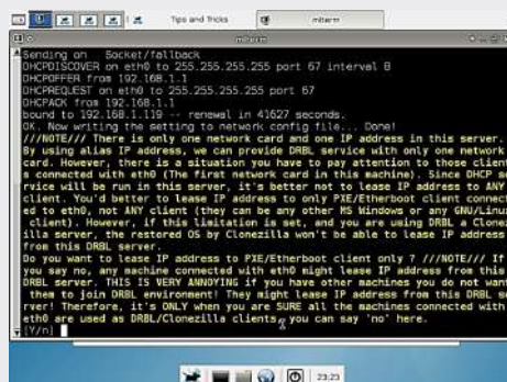
Fig. 3.71. Configuración de red (DHCP)
