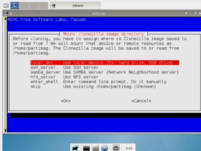
Fig. 3.54. Crear una imagen de un dispositivo (device-image) o clonar directamente desde un disco/partición a otro (device-device)
