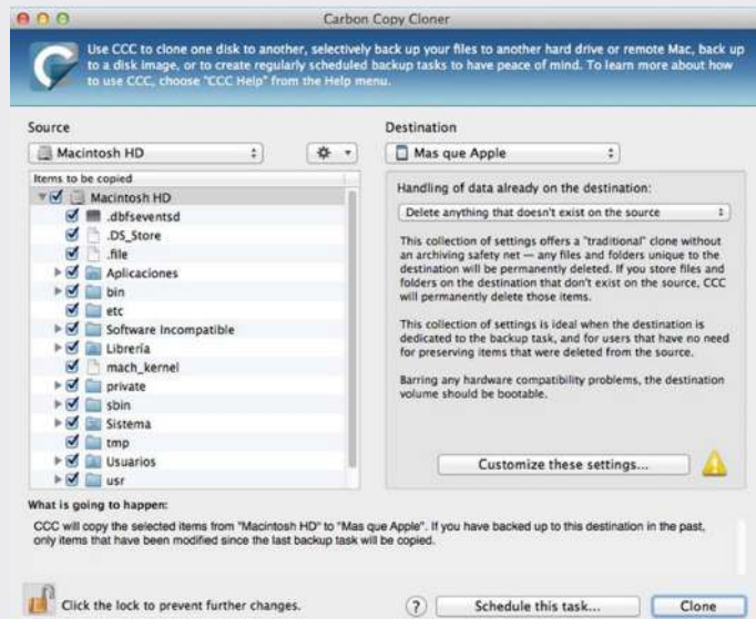
Fig. 3.52. Clonamos el disco
