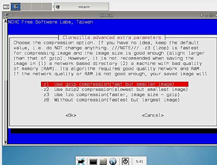
Fig. 3.66. Escojo la opción -Z1 para comprimir la imagen
