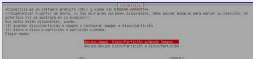
Fig. 3.32. Clonar particiones con la opción device-image
