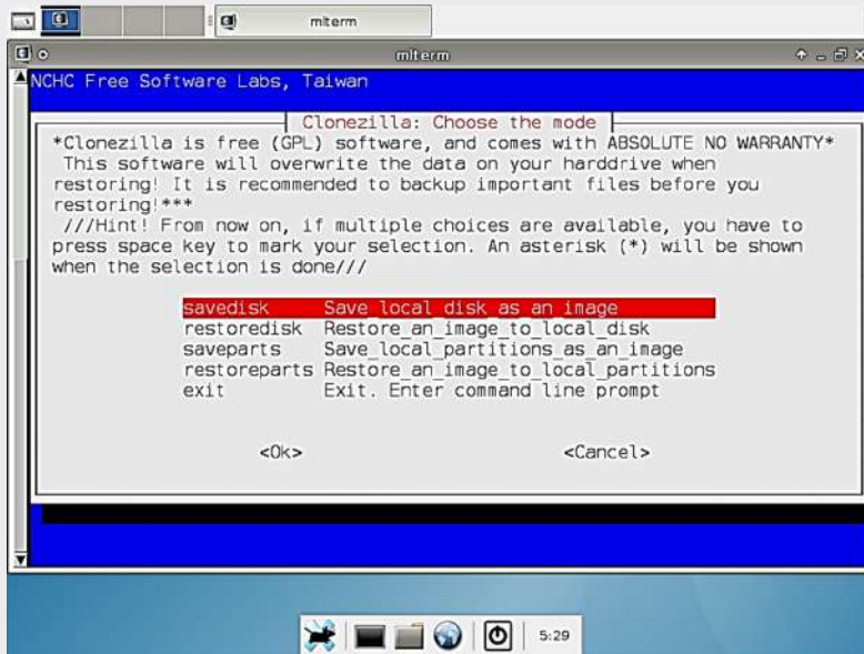
Fig. 3.62. Grabamos la imagen del disco duro local
