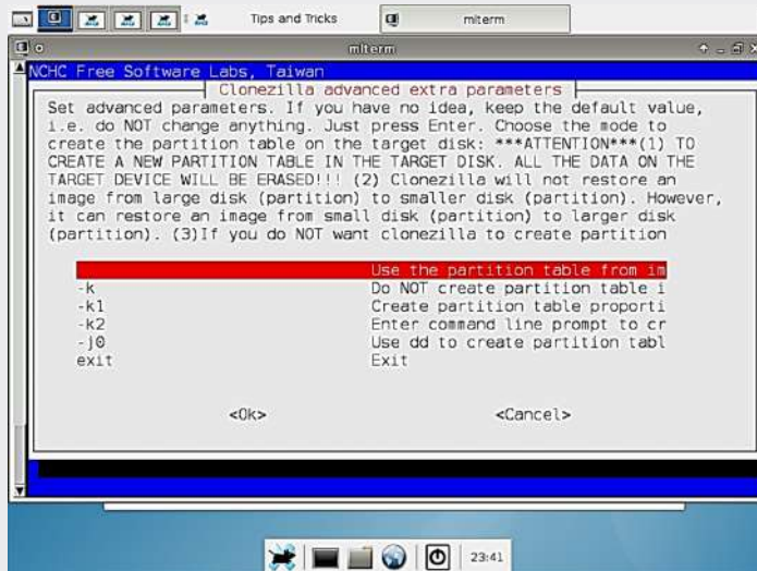
Fig. 3.75. Escogemos usar la tabla de particiones
