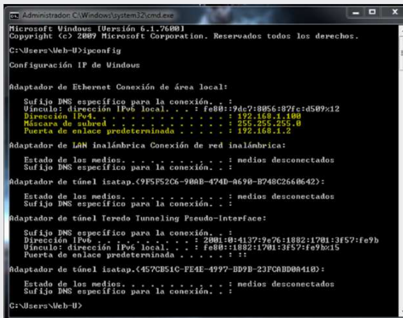
Fig. 3.17. Pantalla con nuestra dirección Ip
