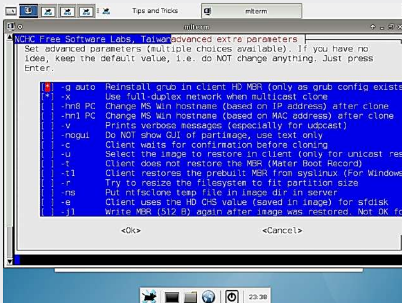
Fig. 3.74. Opciones predeterminadas y continuamos
