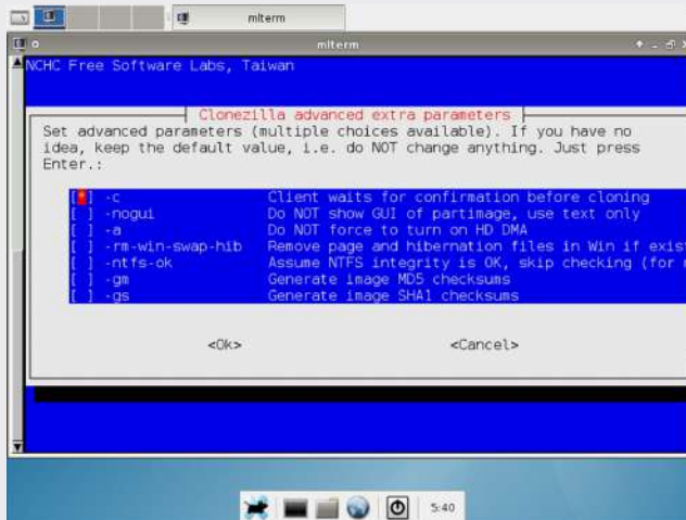
Fig. 3.65. Esperamos la confirmación para clonar nuestro disco duro
