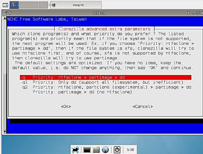
Fig. 3.64. Escogemos la prioridad a grabar
